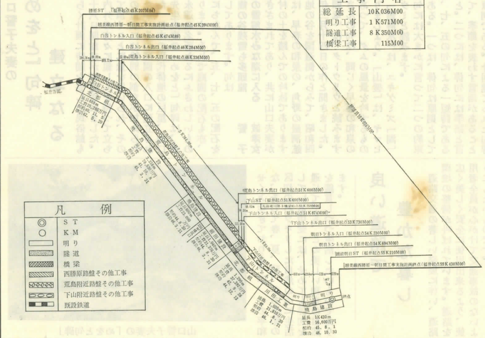
越美線西勝原～朝日間工事施工計画図
