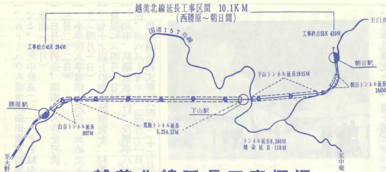
越美北線延長工事概況
