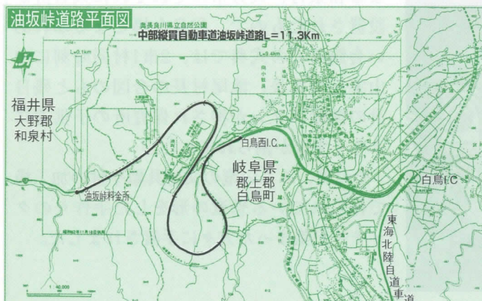
油坂峠道路平面図
