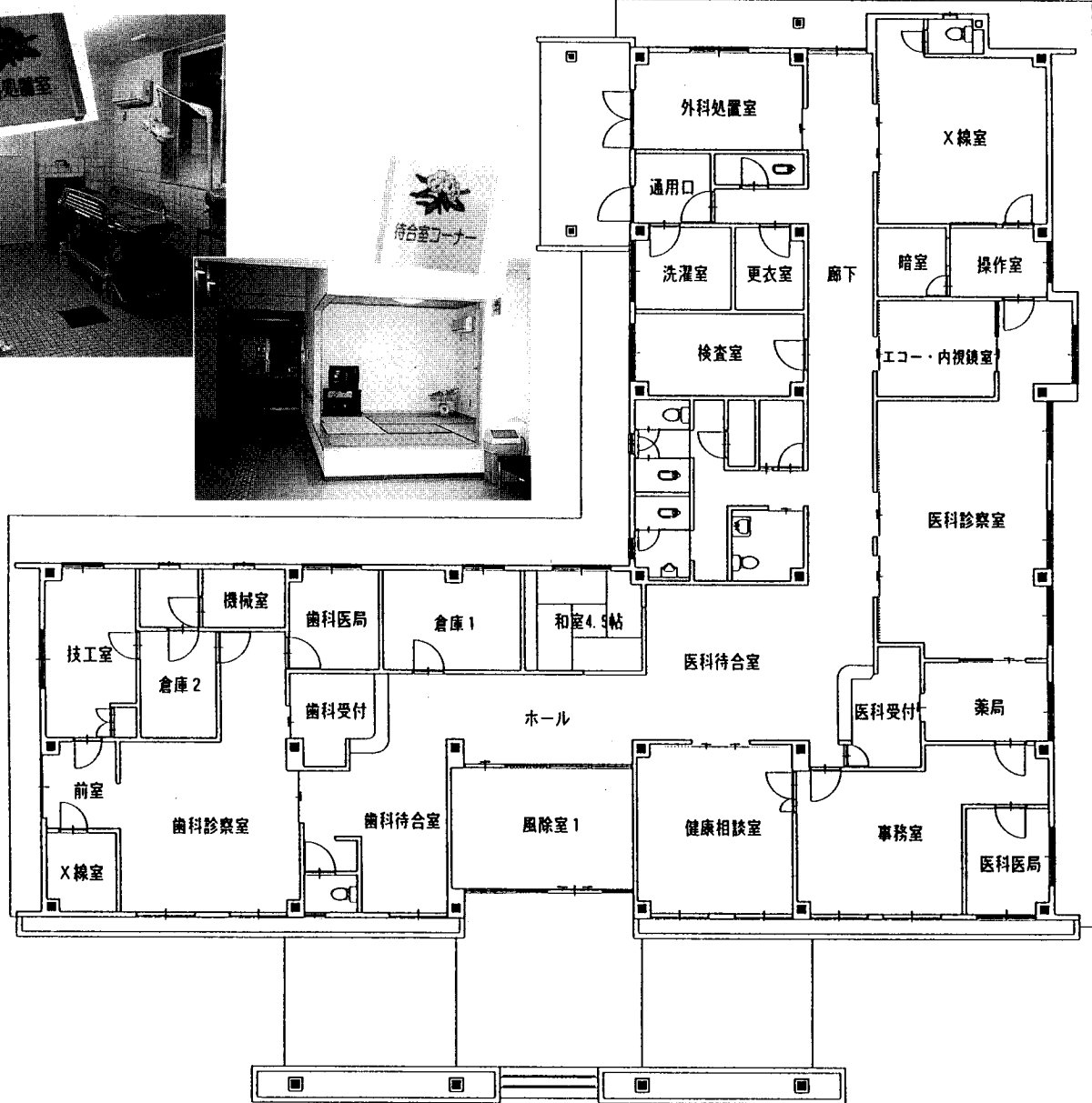
診療所の平面図
